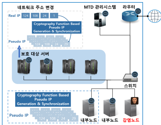
(그림 6) 네트워크 주소 변이 적용 환경
