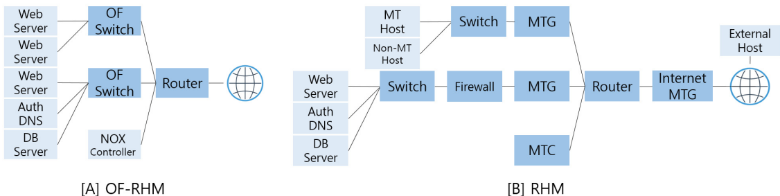
(그림 4) OF-RHM과 RHM의 시스템 아키텍처 개요
