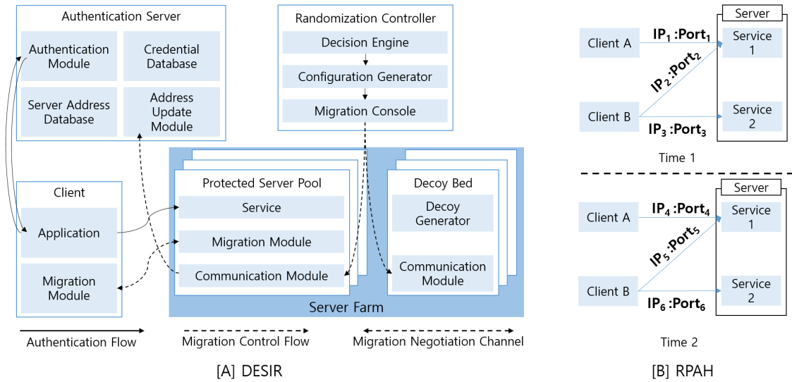
(그림 5) DESIR와 RPAH의 시스템 아키텍처 개요
